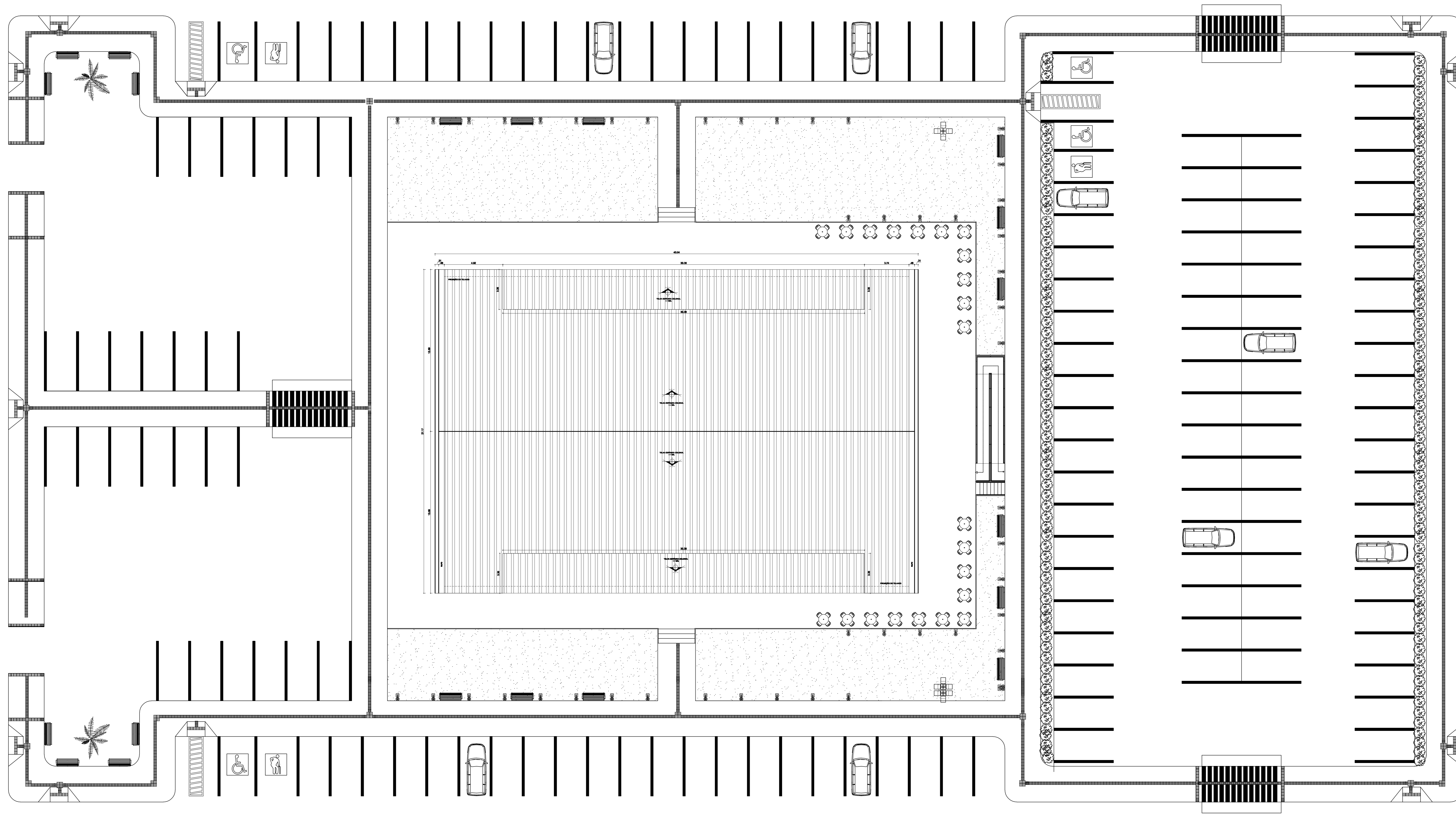
IMPLANTAÇÃO ESC.: 1/125
