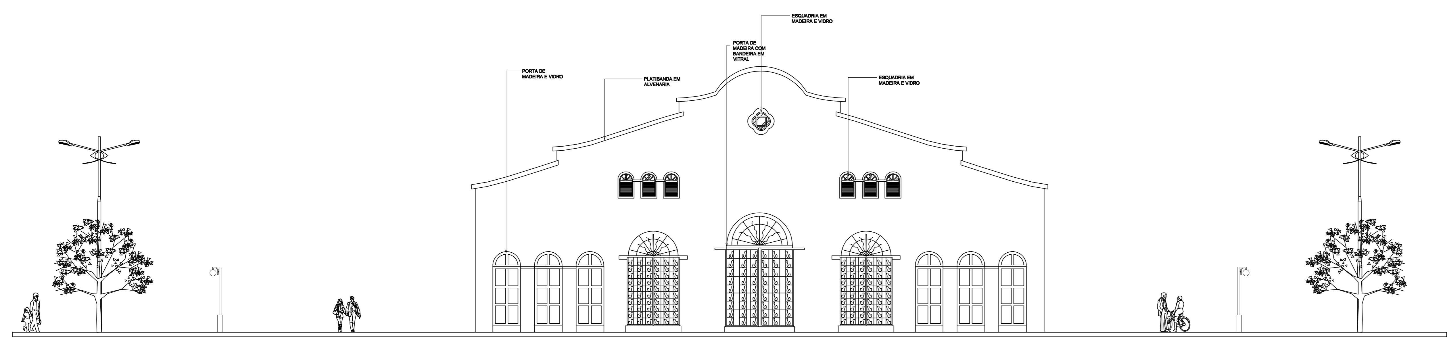
FACHADA PRINCIPAL ESC.: 1/100
