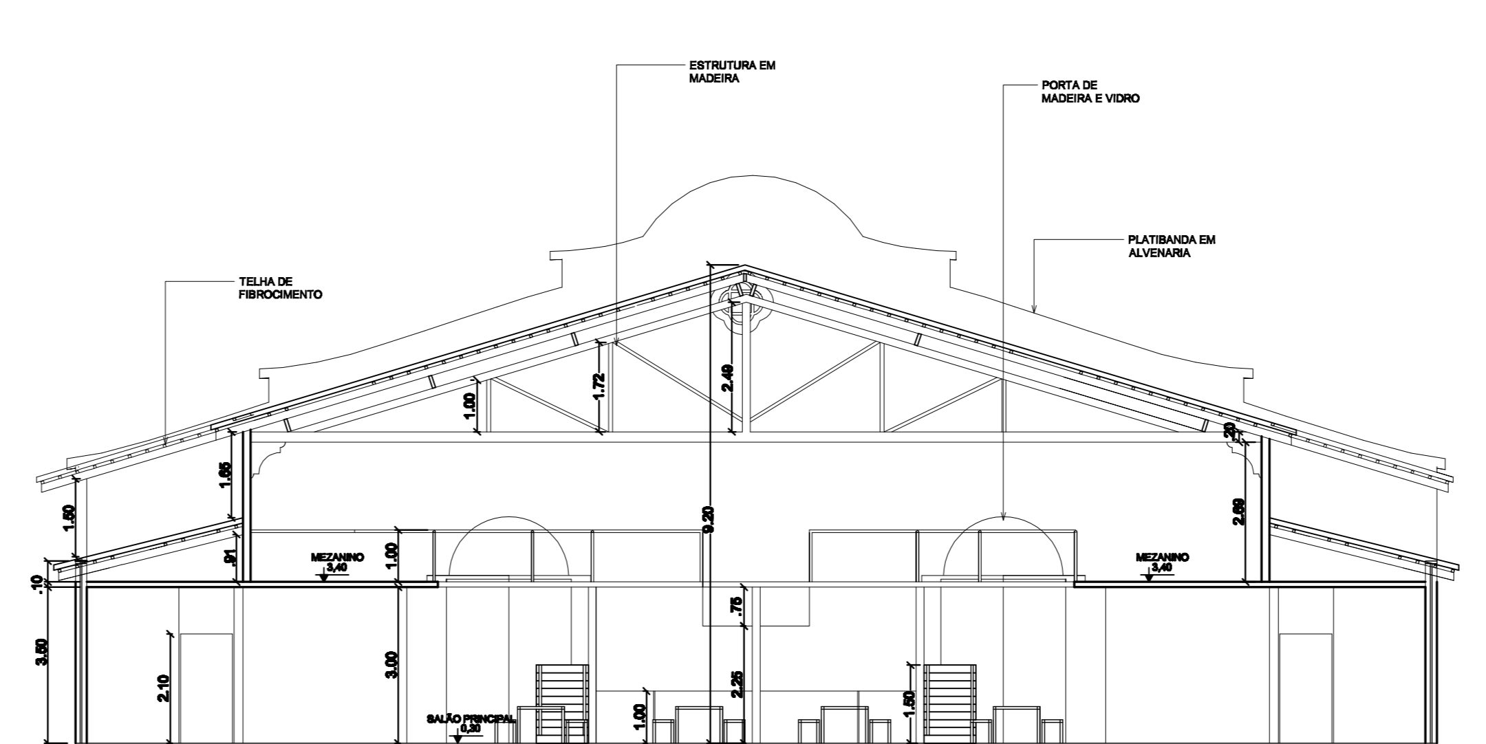
CORTE BB' ESC.: 1/100
