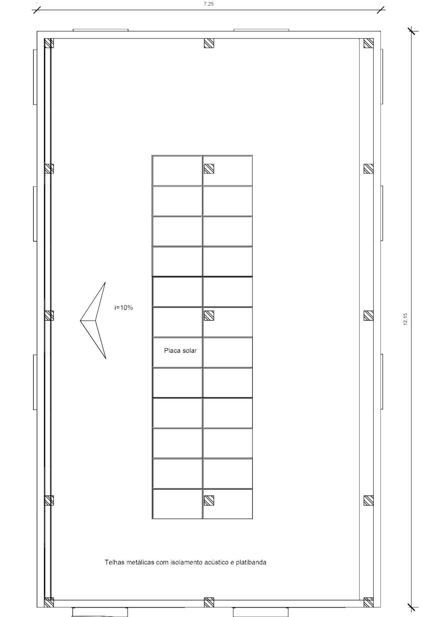
PLANTA DE COBERTURA - VESTIÁRIO esc 1:50
