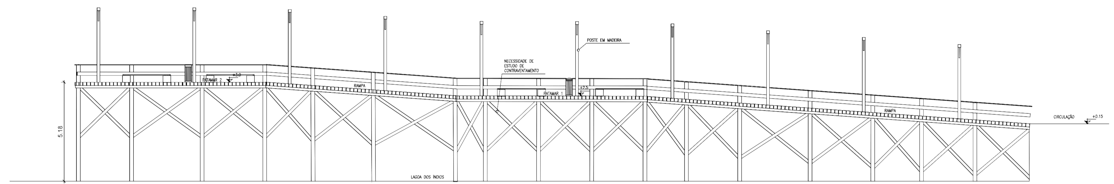
CORTE D - PASSARELA ASCENDENTE COM VÉRTICE esc 1:100
