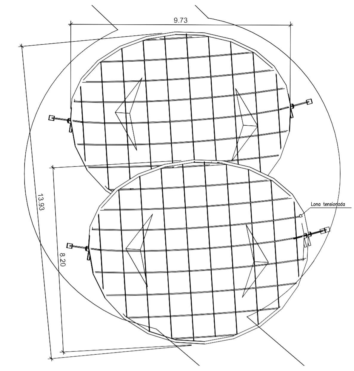
PLANTA DE COBERTURA - GINÁSTICA PARA TERCEIRA IDADE esc 1:100
