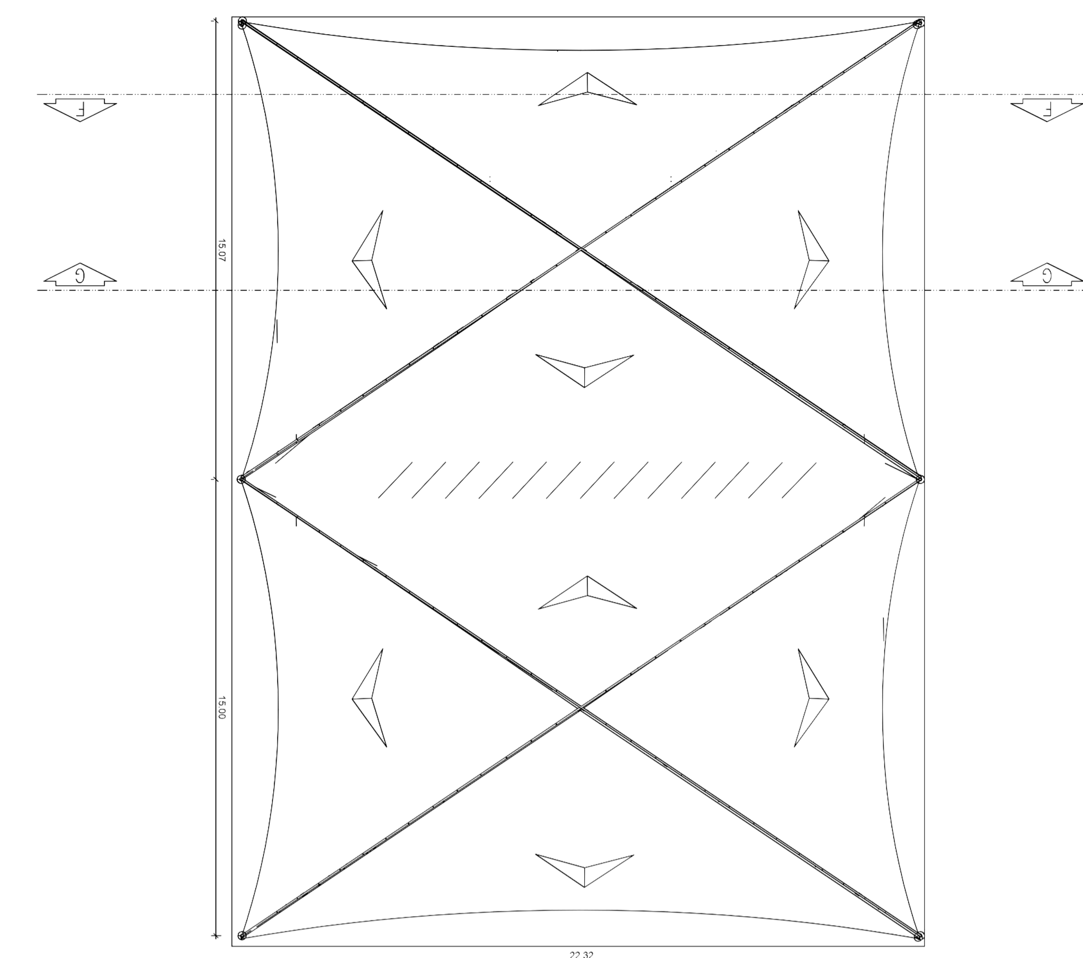
PLANTA DE COBERTURA - BARRACÃO MULTIUSO esc 1:125
