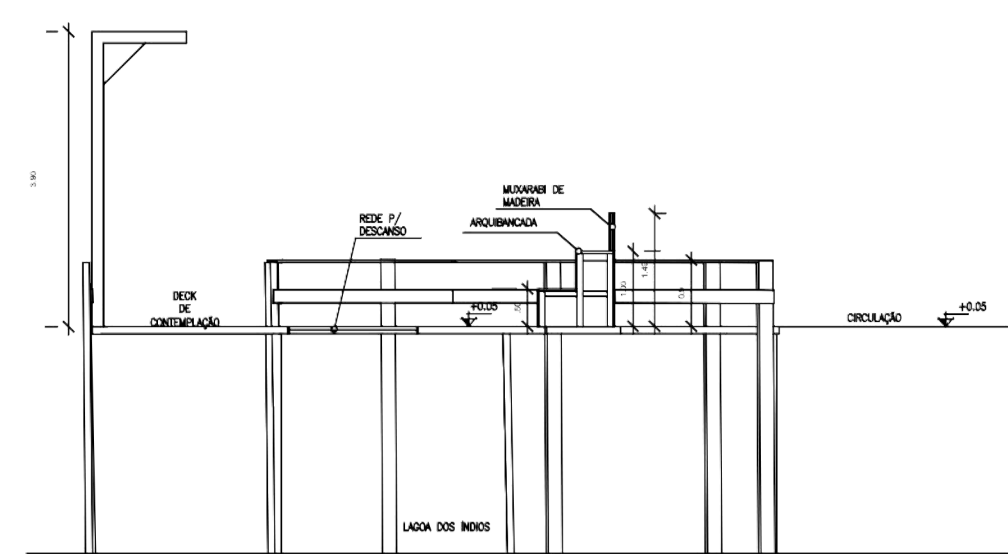
CORTE E - DECK DE CONTEMPLAÇÃO esc 1:100
