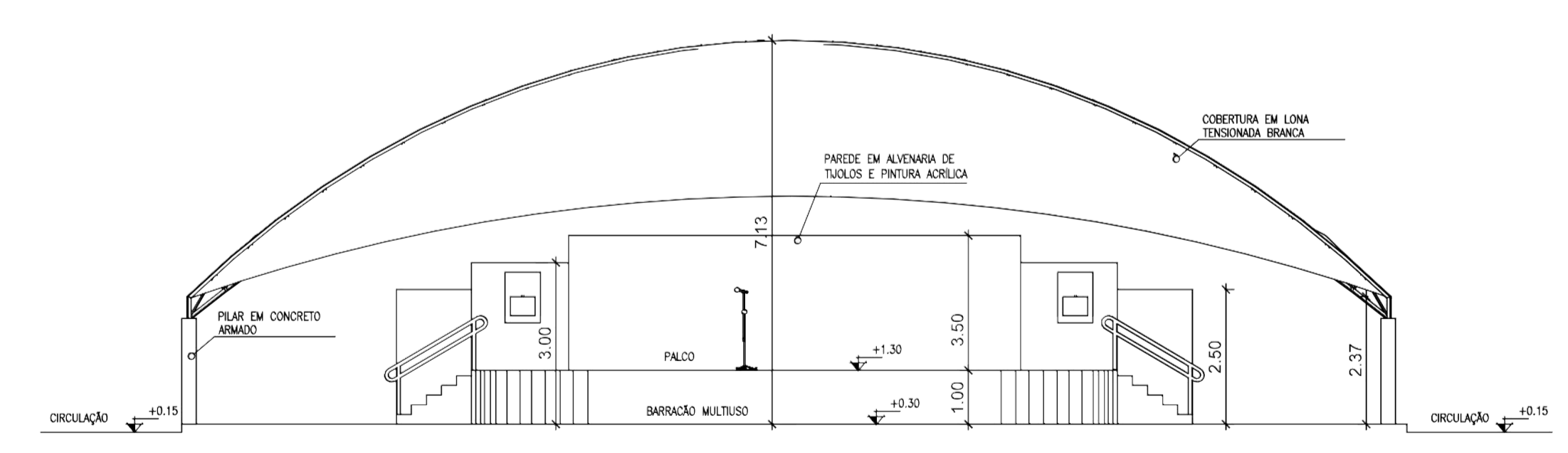
CORTE G - BARRACÃO MULTIUSO esc 1:100
