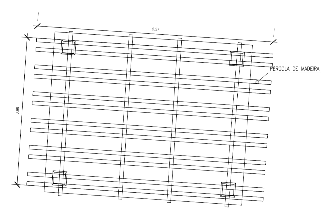
PLANTA DE COBERTURA - RECANTO DE CONTEMPLAÇÃO esc 1:50
