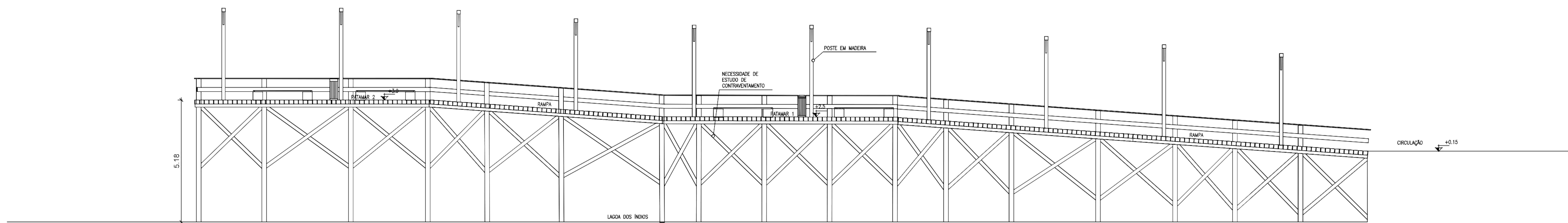
CORTE C - PASSARELA ASCENDENTE esc 1:100
