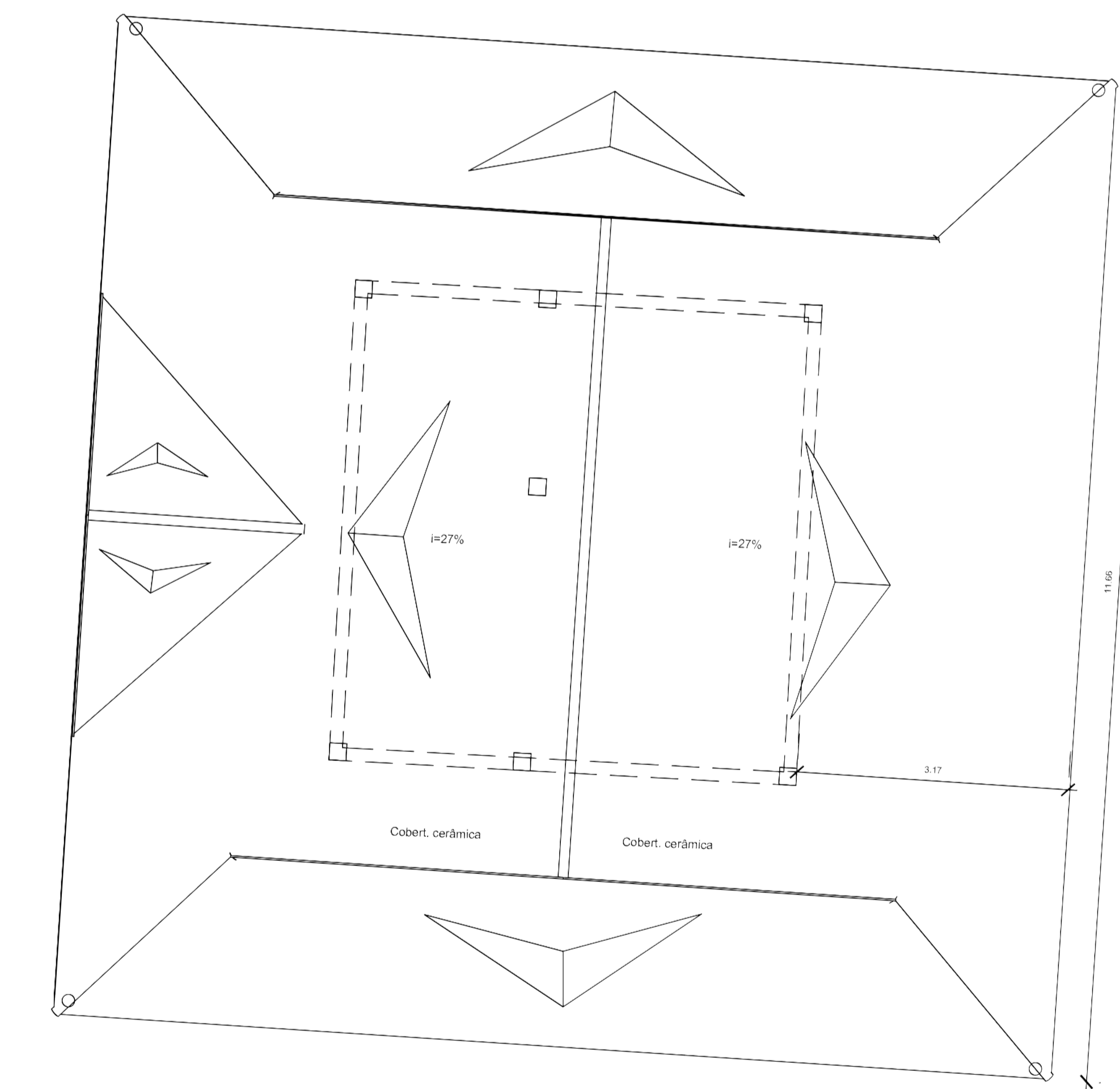
PLANTA DE COBERTURA - LANÇONETE 1 esc 1:50
