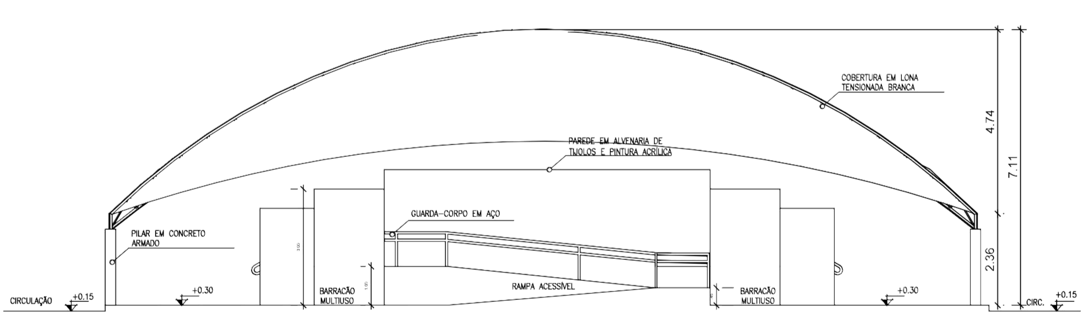
CORTE F - BARRACÃO MULTIUSO esc 1:100
