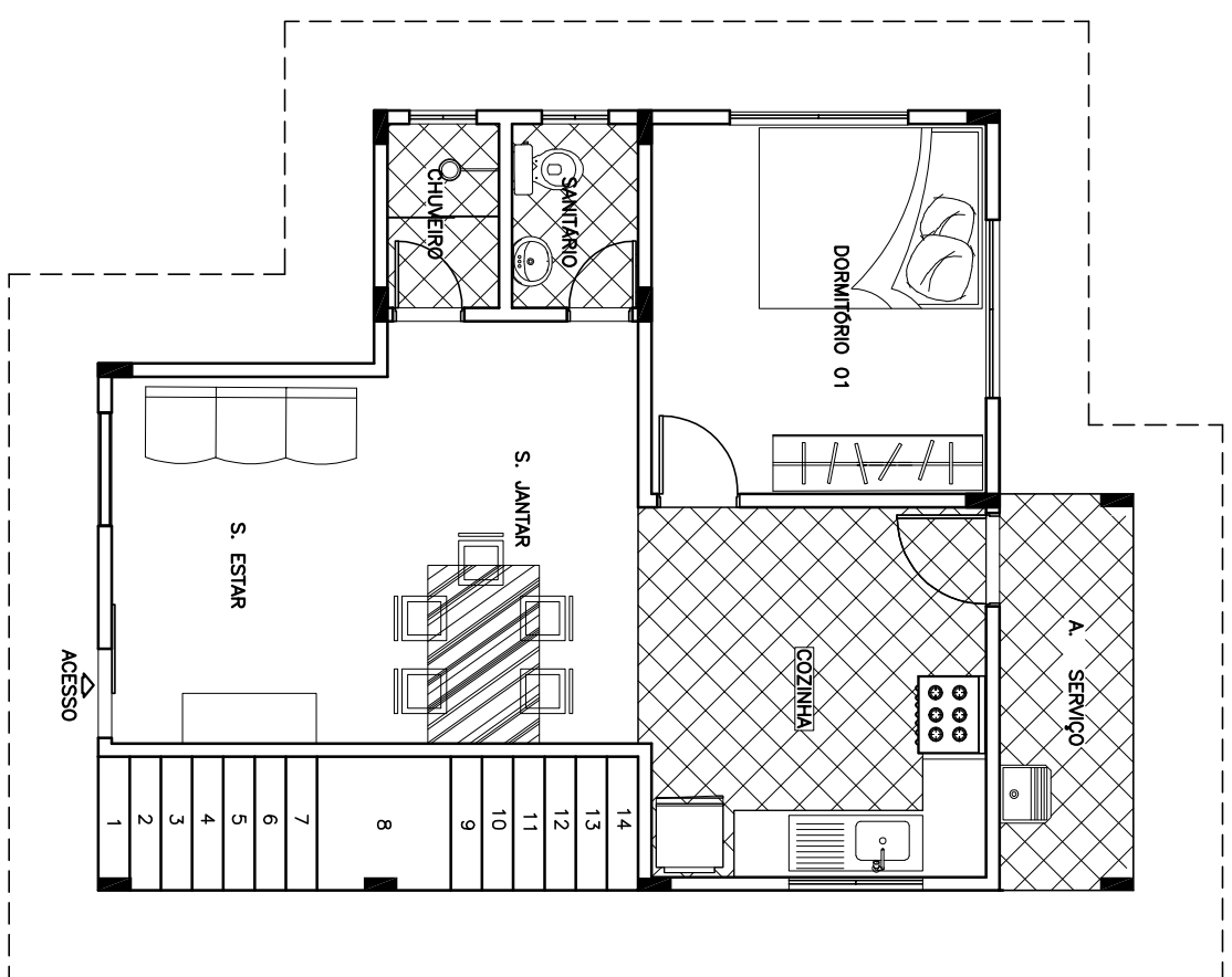
LAYOUT PAV. TÉRREO esc 1:75
