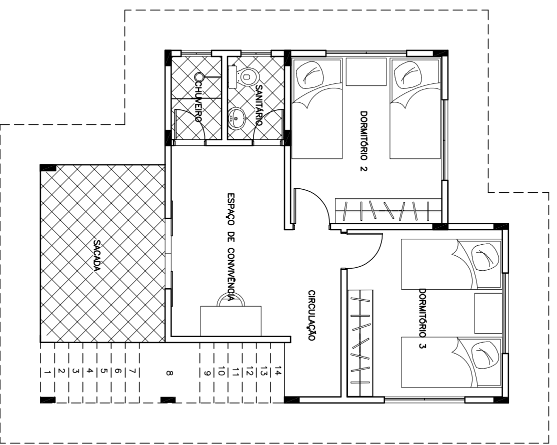
LAYOUT PAV. SUPERIOR esc 1:75
