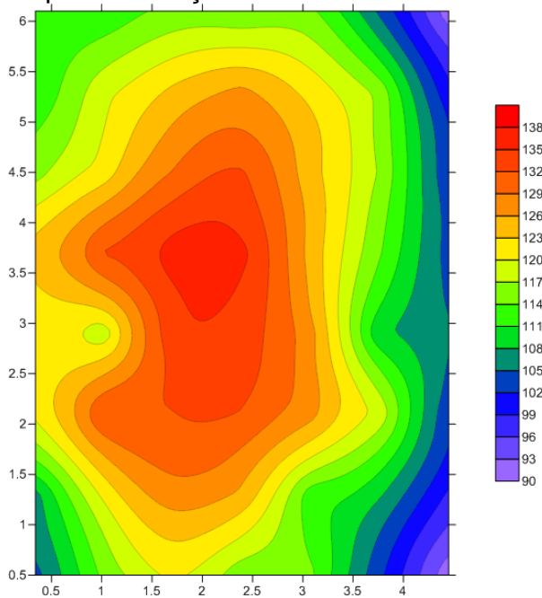
Figura 39 - Gráfico para mediação as 10h da manhã do dia 10/05/2015.
