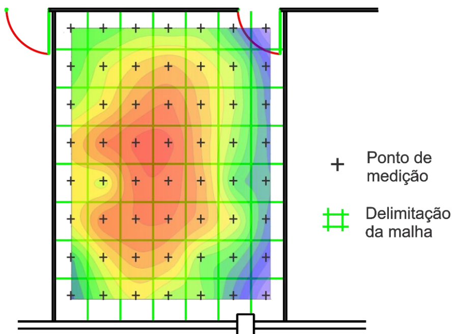
Figura 40 – Sobreposição do gráfico sobre a malha de medição
