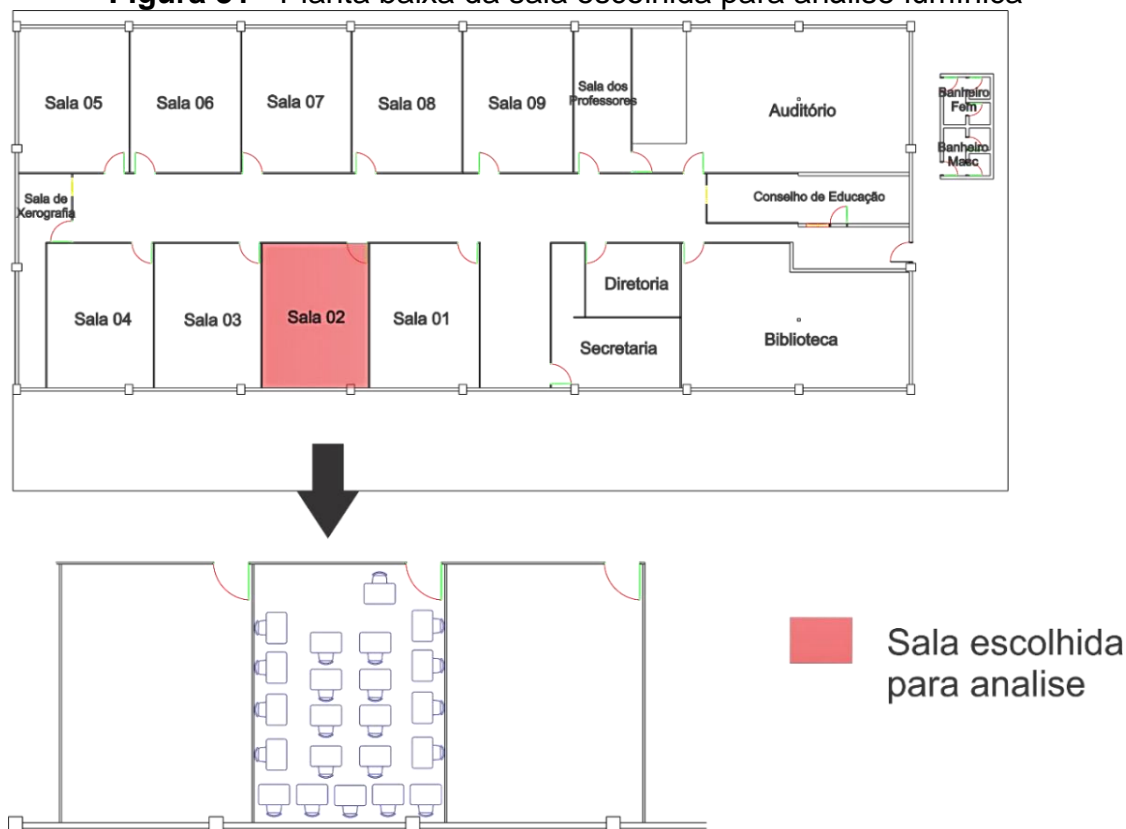
Figura 31 - Planta baixa da sala escolhida para análise lumínica
