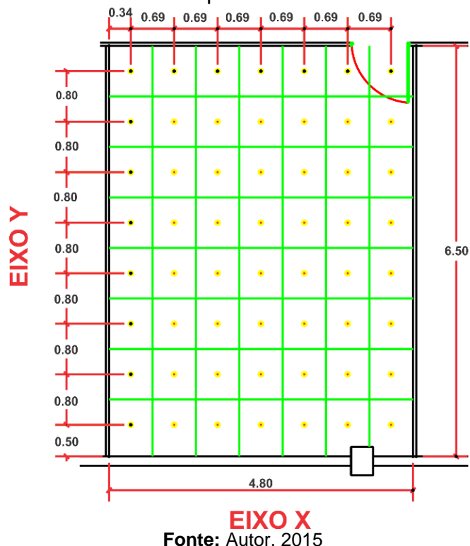
Figura 38 - Planta baixa esquemática com a malha de medição
